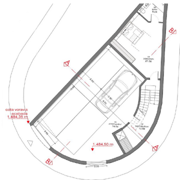
PIANTA CORTESANI
